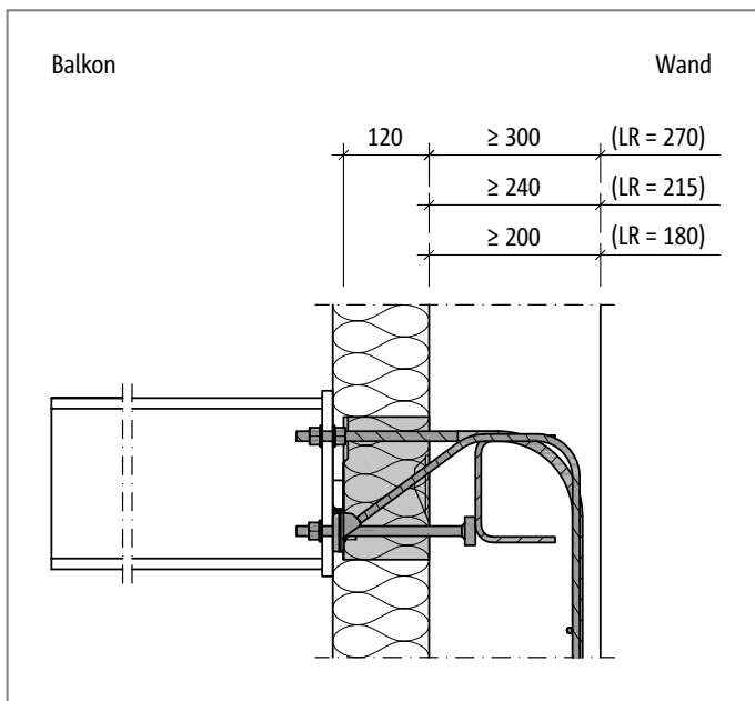
Abb. 13: Schöck Isokorb® XT Typ SK-WU: Sonderkonstruktion für Wandanschluss
