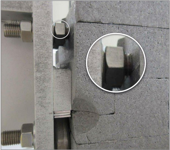
Abb. 52: Innere Mutter an oberen Schrauben zum Einstellen einer Überhöhung
