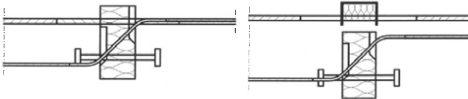
Abb. 1 Schöck Isokorb® Typ K
