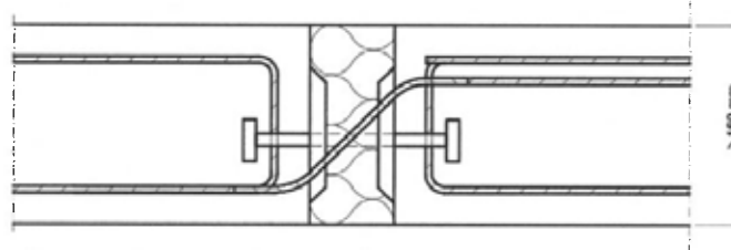
Abb. 19 Beispiel Schöck Isokorb® Typ Q mit SCE und bauseitiger Bewehrung
