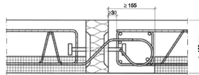
Abb. 29 Beispiel Schöck Isokorb® Typ Q mit Elementplatten
