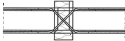
Abb. 6 Schöck Isokorb® Typ D
