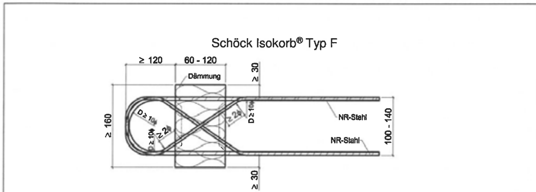
Abb. 25 Schöck Isokorb® Typ F mit SCE
