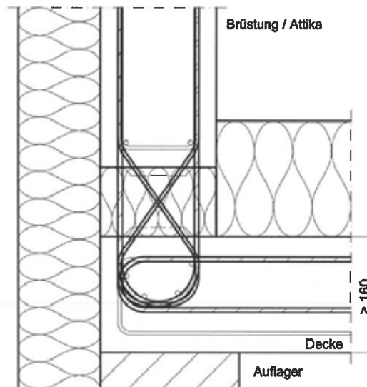
Abb. 24 Beispiel Schöck Isokorb® Typ A mit SCE und bauseitiger Bewehrung
