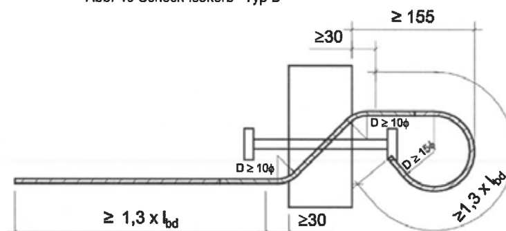
Abb. 41 Schöck Isokorb® Typ Q mit und ohne Randbalken
