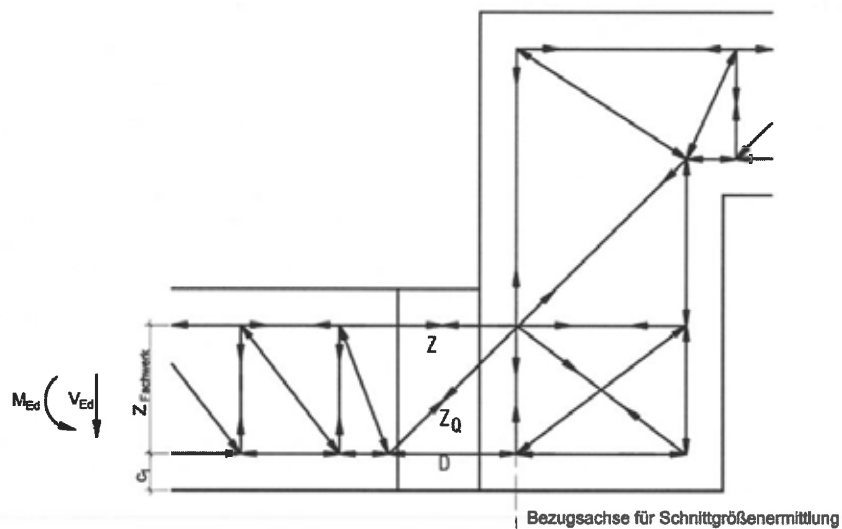
Abb. 35 Schöck Isokorb® Typ K (Variante Höhenversatz)
