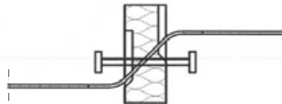
Abb. 4 Schöck Isokorb® Typ Q
