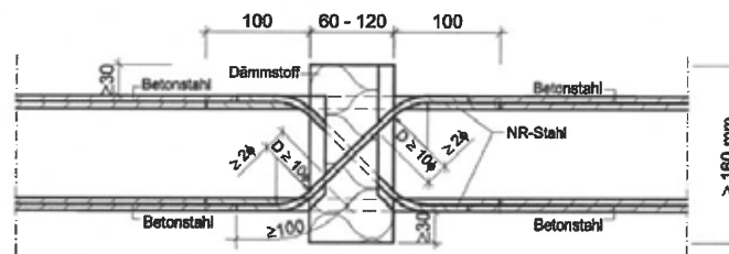
Abb. 21 Schöck Isokorb® Typ D mit SCE
