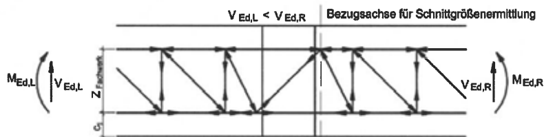
Abb. 38 Schöck Isokorb® Typ D (Typ A und F analog)
