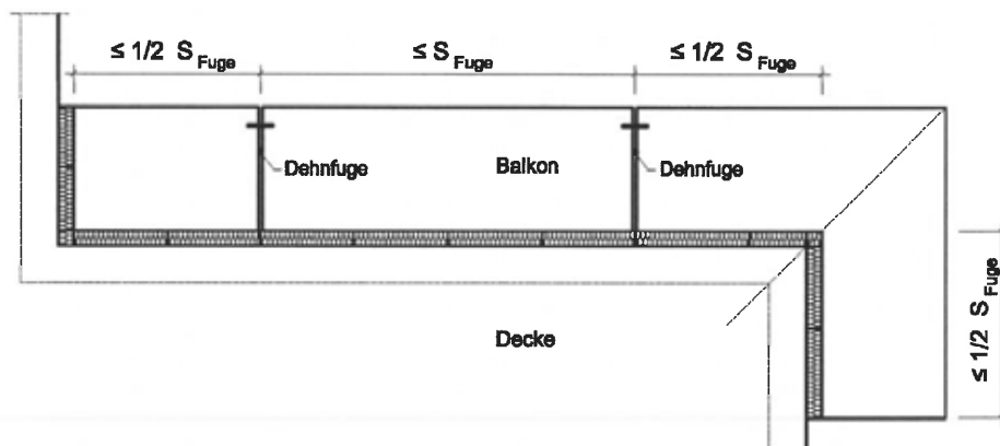
Abb. 12 Einbausituation mit Dehnfugen
