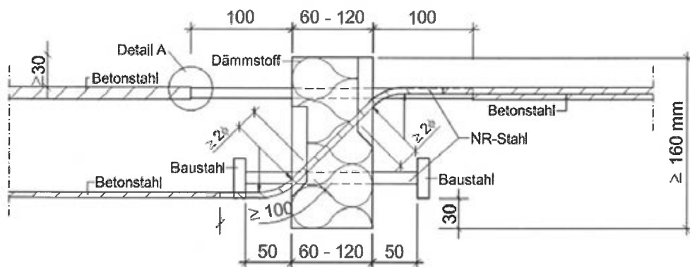
Abb. 9 Schöck Isokorb® K mit SCE
