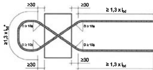
Abb. 42 Schöck Isokorb® Typ A
