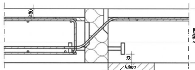
Abb. 15 Beispiel Schöck Isokorb® Typ K mit SCE und bauseitiger Bewehrung
