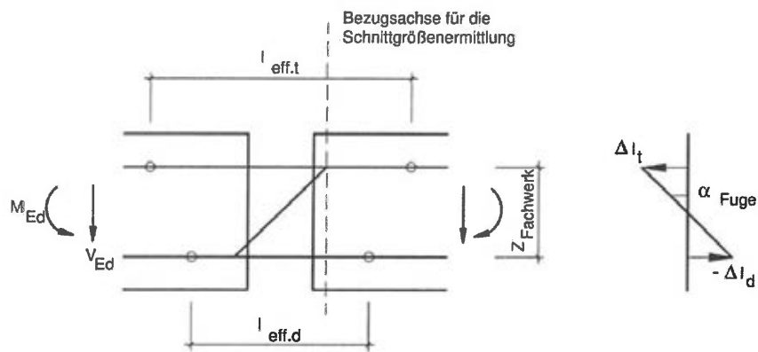
Abb. 47 Modell für die Ermittlung der Biegeverformung in der Fuge
