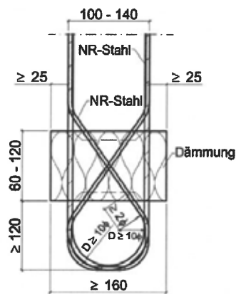
Abb. 23 Schöck Isokorb® Typ A mit SCE
