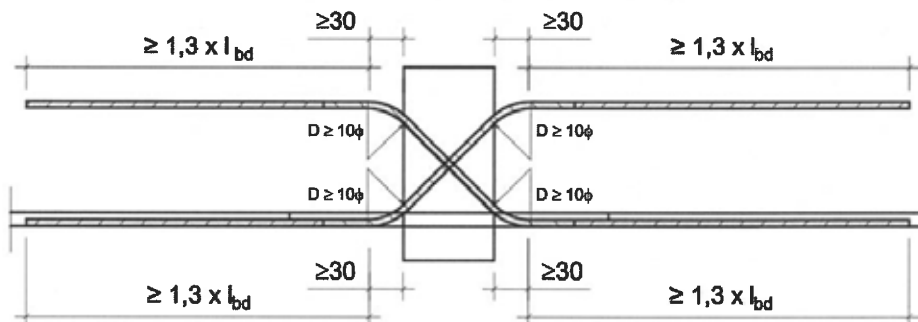
Abb. 40 Schöck Isokorb® Typ D
