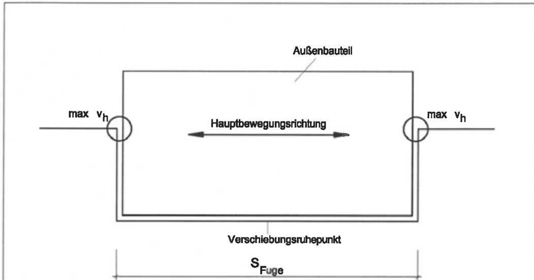
Abb. 11 Einbausituation mit Lagerung zwischen gegenüberliegenden Rändern
