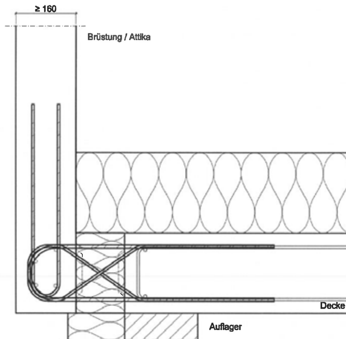
Abb. 26 Beispiel Schöck Isokorb® Typ F mit SCE und bauseitiger Bewehrung
