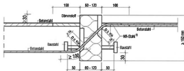
Abb. 13 Schöck Isokorb® Typ K mit SCE
