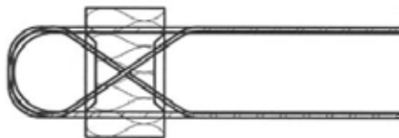
Abb. 7 Schöck Isokorb® Typ A
