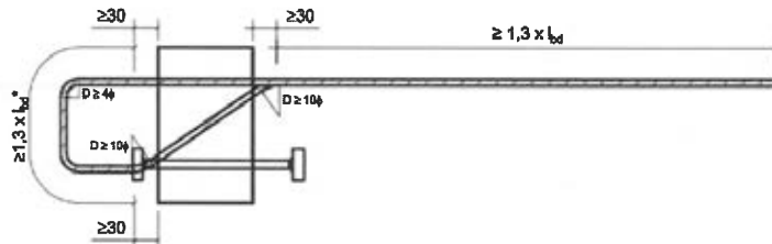
Abb. 44 Schöck Isokorb® Typ O
