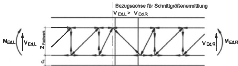
Abb. 37 Schöck Isokorb® Typ D (Typ A und F analog)
