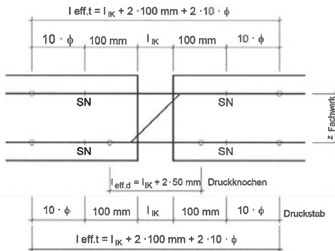
Abb. 49 l_{eff} für nichtrostenden glatten Stabstahl Fkl. S 355, S 460 und S 690 gem. Abschn. A.3
