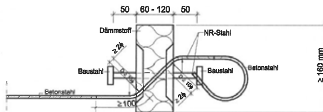
Abb. 45 Schöck Isokorb® Typ Q mit SCE
