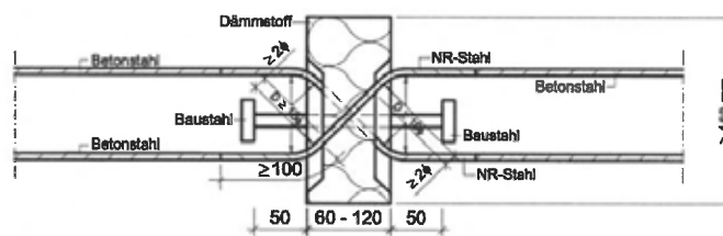
Abb. 20 Schöck Isokorb® Typ Q+Q mit SCE
