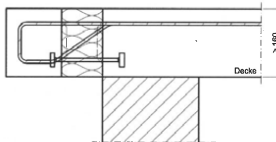
Abb. 17 Beispiel Schöck Isokorb® Typ O mit SCE
