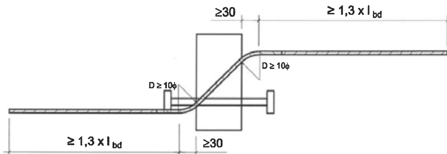
Abb. 39 Schöck Isokorb® Typ K/KF (Variante mehrteilig)
