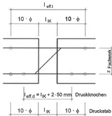
Abb. 48 l_{eff} für nichtrostenden gerippten Stabstahl gem. Abschn. A.3
