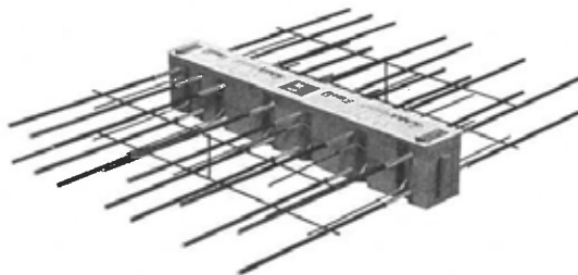
Abb. 5 Schöck Isokorb® Typ D
