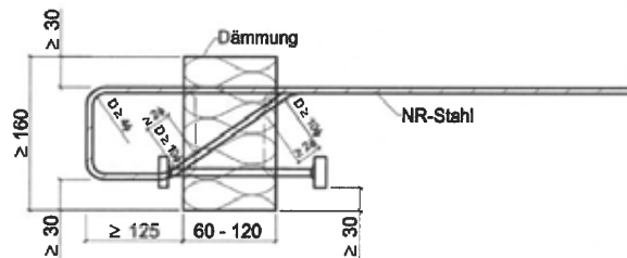
Abb. 16 Schöck Isokorb® Typ O mit SCE
