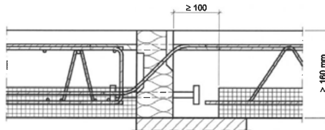
Abb. 27 Beispiel Schöck Isokorb® Typ K und KF (Variante mehrteilig) mit Elementplatten
