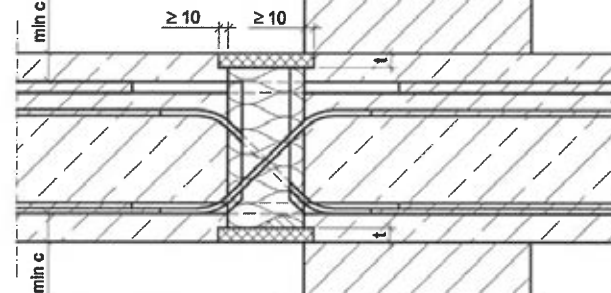
Abb. 31 Schöck Isokorb® Typ D (analog A und F) mit SCE
