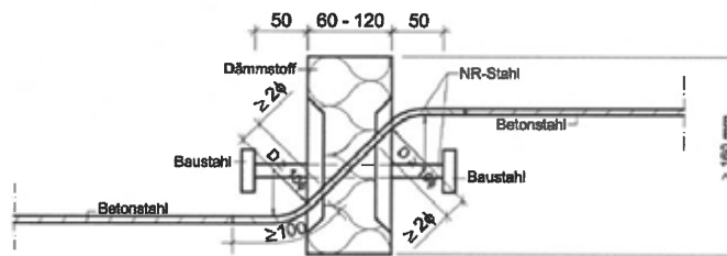
Abb. 18 Schöck Isokorb® Typ Q mit SCE
