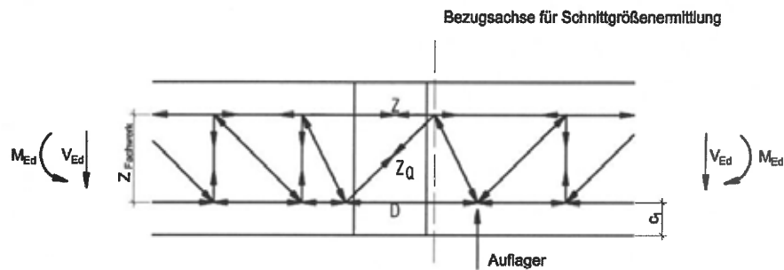
Abb. 34 Schöck Isokorb® Typ K und KF (Variante mehrteilig) (Typ O analog)
