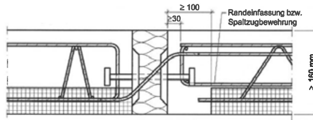
Abb. 28 Beispiel Schöck Isokorb® Typ Q mit Elementplatten
