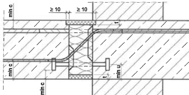
Abb. 30 Schöck Isokorb® Typ K und KF (analog O) mit SCE
