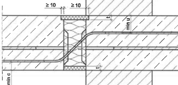
Abb. 32 Schöck Isokorb® Typ Q und Typ QF
