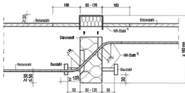
Abb. 14 Schöck Isokorb® Typ KF (Variante mehrteilig) mit SCE
