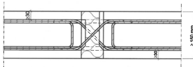
Abb. 22 Beispiel Schöck Isokorb® Typ D mit SCE und bauseitiger Bewehrung
