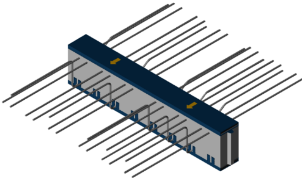
Abbildung 2: Schöck Isokorb® XT Typ K-M4-V2-REI120-CV50-X120-H220-L1000-6.0
