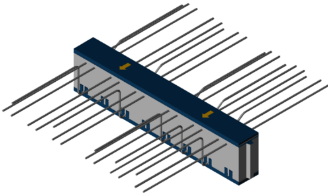
Abbildung 2: Schöck Isokorb® XT Typ K-M4-V2-REI120-CV35-X120-H220-L1000-6.0
