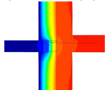
Isothermenbild des XT Typ K-M6V2
