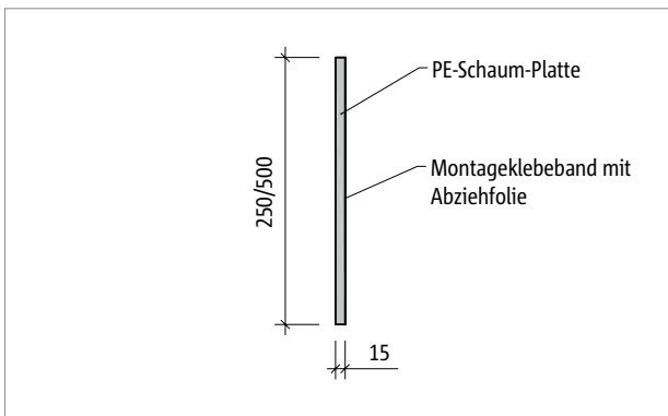
Abb. 185: Schöck Tronsole® Typ L: Produktschnitt
