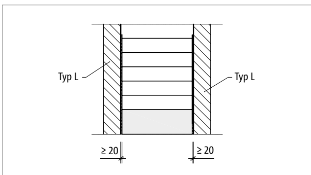
Abb. 187: Schöck Tronsole® Typ L: Berücksichtigung von Einbautoleranzen
