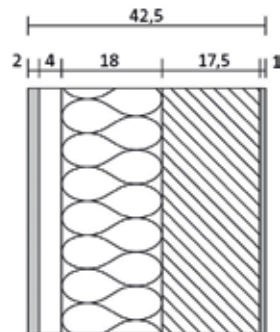
Wandaufbau mit 3 Edelstahlwandhaltern und 18 cm Mineralwolle WL 035
