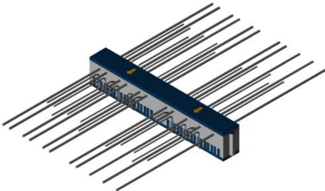
Abbildung 2: Schöck Isokorb® XT Typ K-M8-VV1-REI120-CV35-X120-H180-L1000-6.0
