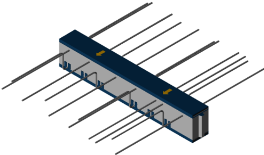
Abbildung 2: Schöck Isokorb® XT Typ K-M2-V2-REI120-CV35-X120-H180-L1000-6.0
