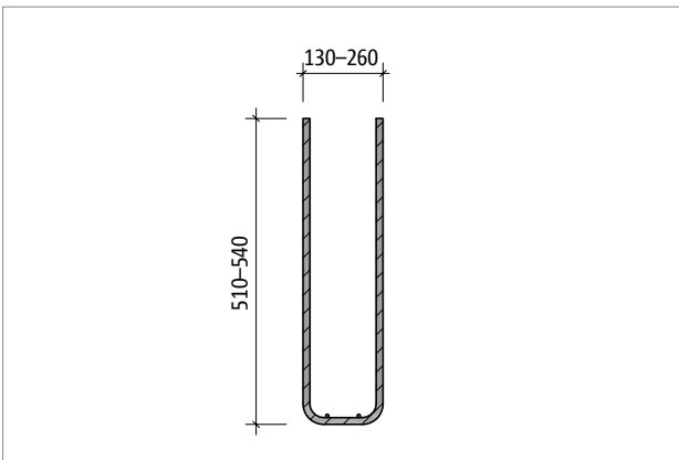
Abb. 199: Schöck Sconnex® Typ W Part TB: Zulagebewehrung 3 \varnothing 12/65 mm; Bügel als Spaltzugbewehrung
