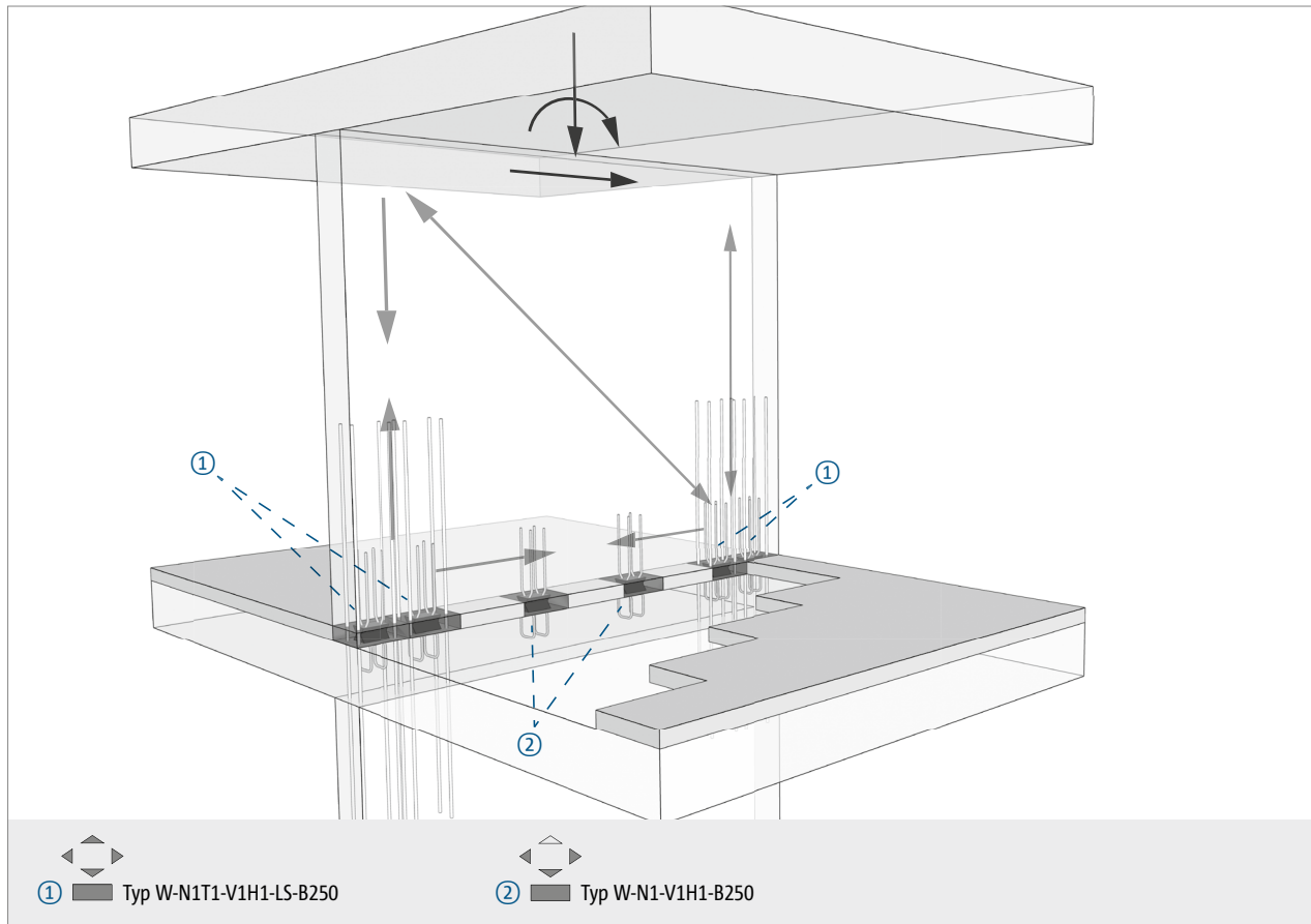
Abb. 157: Gebäudestabilisierende Wand auf Decke getrennt
