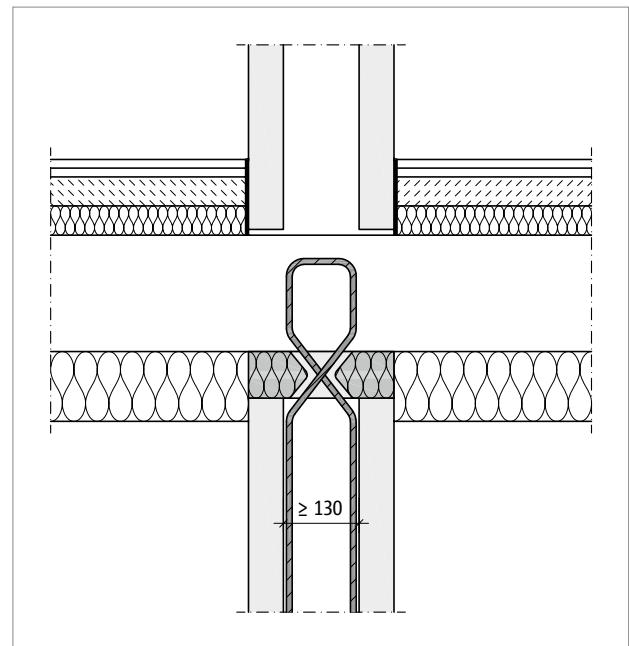
Abb. 240: Schöck Sconnex® Typ W: Schematische Darstellung Schöck Sconnex® Typ W bei Doppelwänden und Unterdeckendämmung
