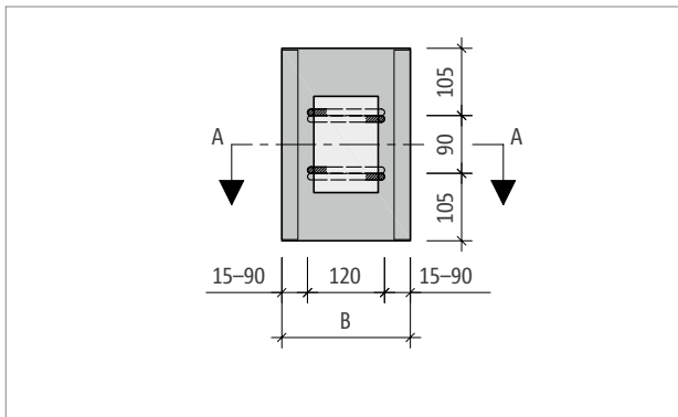
Abb. 175: Schöck Sconnex® Typ W-N-VH: Produktgrundriss; Positionierung der Querkraftstäbe
