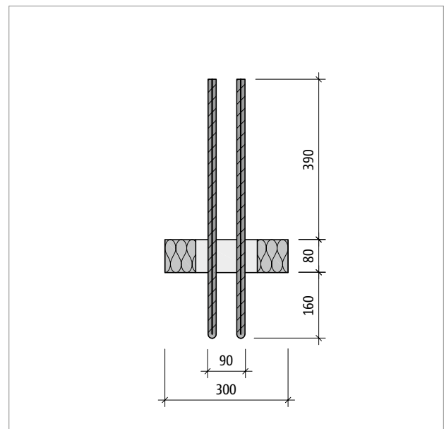
Abb. 178: Schöck Sconnex® Typ W-N-VH: Produktschnitt B-B
