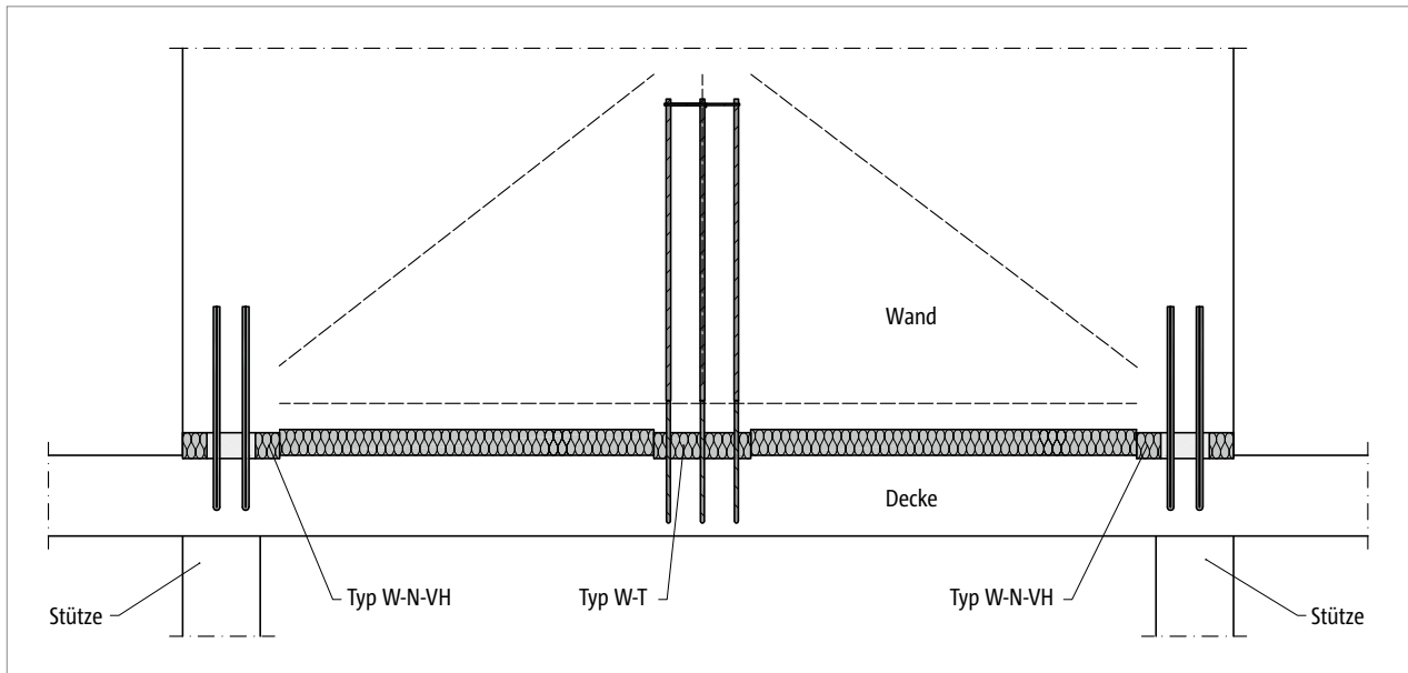
Abb. 142: Schöck Sconnex® Typ W: Kombinierte Produktvarianten für den Anschluss eines wandartigen Trägers mit Deckenaufhängung
