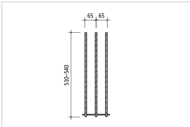
Abb. 200: Schöck Sconnex® Typ W Part TB: Zulagebewehrung 3 \varnothing 12/65 mm; Bügel in der Seitenansicht
