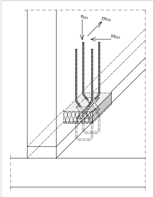
Abb. 245: Schöck Sconnex® Typ W-N-VH: Statisches System
