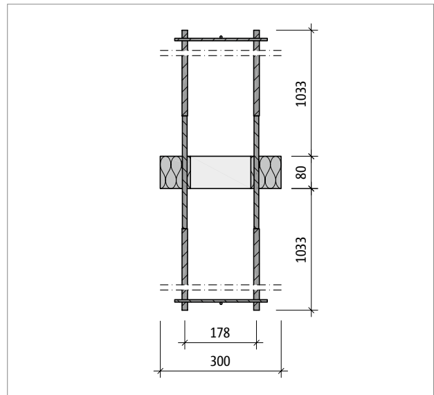
Abb. 184: Schöck Sconnex® Typ W-N1T1-LW: Produktschnitt B-B
