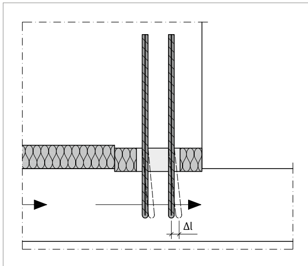
Abb. 172: Schöck Sconnex® Typ W: Verschiebung der äußeren Stäbe um \Delta l infolge einer Temperaturverformung bei Aufdeckendämmung im Detail
