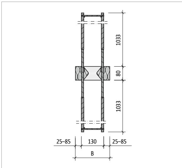
Abb. 183: Schöck Sconnex® Typ W-N1T1-LW: Produktschnitt A-A
