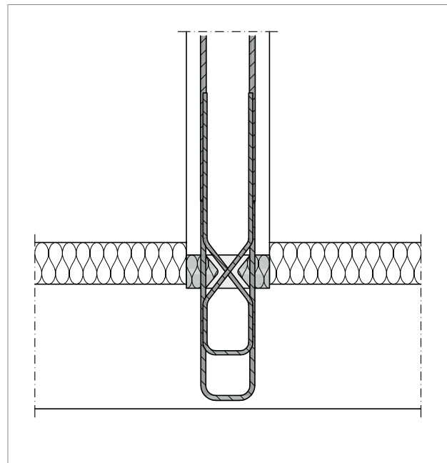
Abb. 146: Schöck Sconnex® Typ W-NT-VH-B: Schnitt E-E; Aufhängung der Decke an eine Wand
