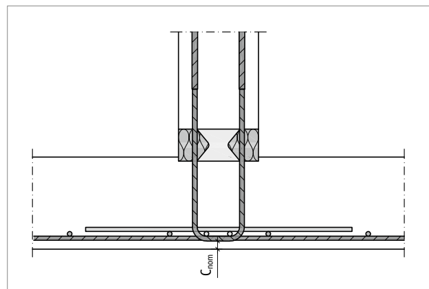
Abb. 163: Schöck Sconnex® Typ W-N1T1-BW: Die zweite Bewehrungslage ist in den Schöck Sconnex® Bügel eingefädelt
