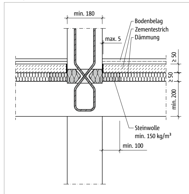
Abb. 202: Schöck Sconnex® Typ W-N-VH: Mit Randstreifen aus Steinwolle im Bereich der Trittschalldämmung
