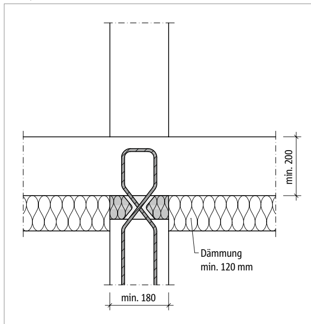
Abb. 207: Schöck Sconnex® Typ W-N-VH: Bei Unterdeckendämmung ohne Brandschutzmaßnahmen
