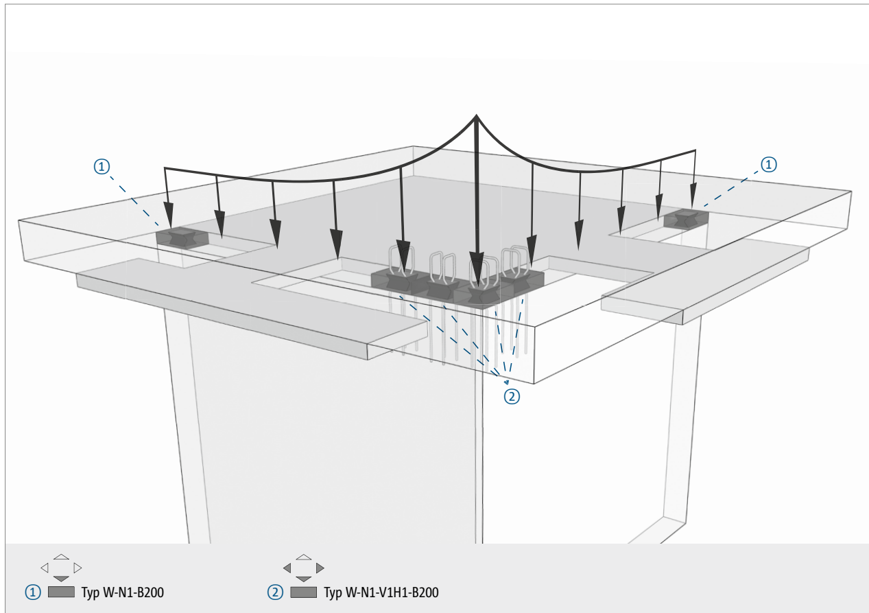
Abb. 151: Wanddecke unter Decke getrennt
