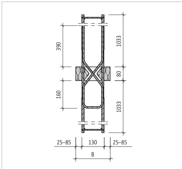
Abb. 189: Schöck Sconnex® Typ W-N1T1-V1H1-LW: Produktschnitt A-A
