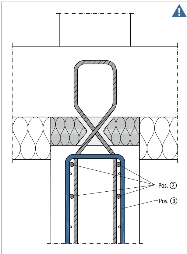
Abb. 234: Schöck Sconnex® Typ W-N-VH: Bauseitige Bewehrung Variante A; der außenliegende Stabstahl Pos. 2 stützt die Querkraftstäbe des Schöck Sconnex® gegen die Bauteiloberfläche ab
