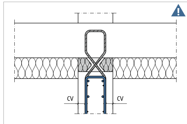
Abb. 166: Schöck Sconnex® Typ W-N-VH: Variante B (für geringe Wanddicken) – bauseitige Bewehrung; die Längsbewehrung stützt die Querkraftstäbe des Schöck Sconnex® gegen das Innere des Stahlbetonbauteils ab
