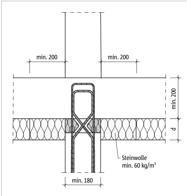
Abb. 219: Schöck Sconnex® Typ W-NT-VH: Mit Randstreifen aus Steinwolle im Bereich der Unterdeckendämmung; Feuerwiderstandsklasse abhängig von der Dicke des Randstreifens
