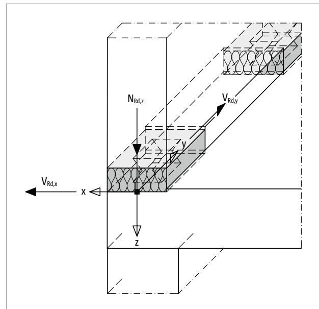
Abb. 168: Schöck Sconnex® Typ W: Vorzeichenregel für die Bemessung
