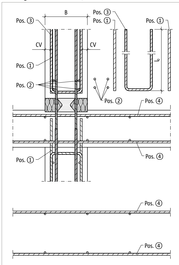
Abb. 226: Schöck Sconnex® Typ W-NT-LW: Bauseitige Bewehrung bei Zugkraftverankerung
