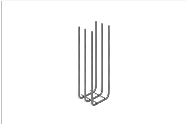
Abb. 150: Schöck Sconnex® Typ W Part TB
