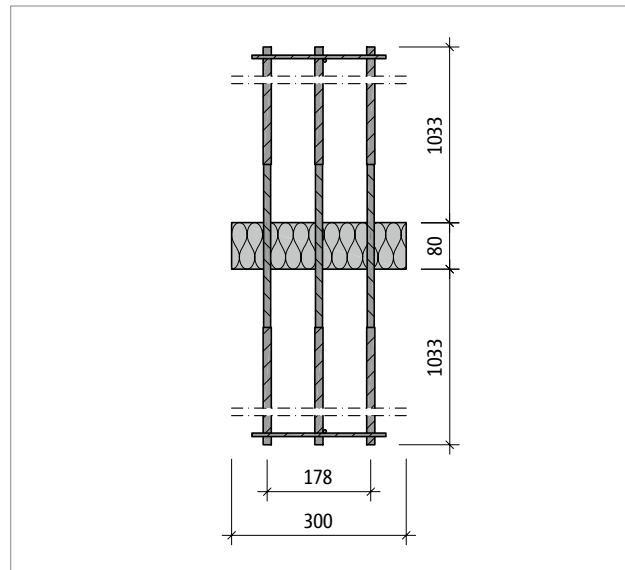
Abb. 196: Schöck Sconnex® Typ W-T1-LW: Produktschnitt B-B
