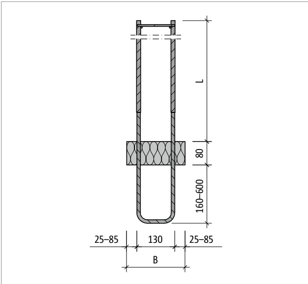
Abb. 193: Schöck Sconnex® Typ W-T2-BW: Produktschnitt A-A
