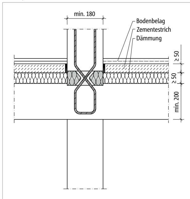
Abb. 201: Schöck Sconnex® Typ W-N-VH: Bei Trittschalldämmung aus EPS
