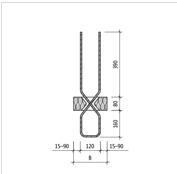
Abb. 177: Schöck Sconnex® Typ W-N-VH: Produktschnitt A-A
