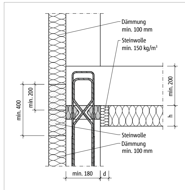
Abb. 223: Schöck Sconnex® Typ W-NT-VH: Bei brennbarem WDVS mit Brandriegel (außen) und Brandschutzstreifen aus Steinwolle (innen); Feuerwiderstandsklasse abhängig von Höhe und Dicke des Brandschutzstreifens
