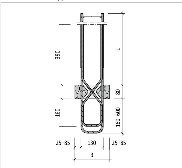
Abb. 187: Schöck Sconnex® Typ W-N1T1-V1H1-BW: Produktschnitt A-A
