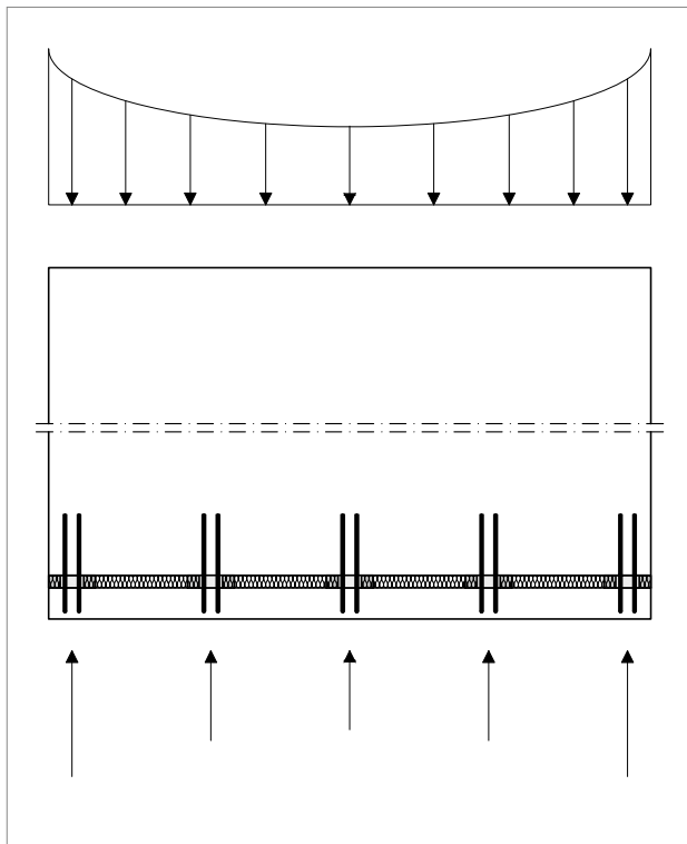
Abb. 134: Schöck Sconnex® Typ W: Parabelförmige Streckenlast - unterschiedliche Kräfte bei gleichen Abständen
