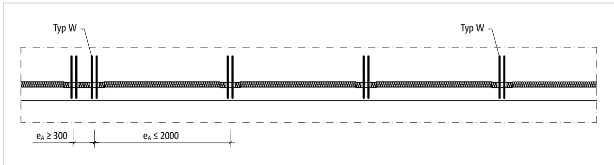
Abb. 169: Schöck Sconnex® Typ W: Minimaler und maximaler Achsabstand e_A [mm]
