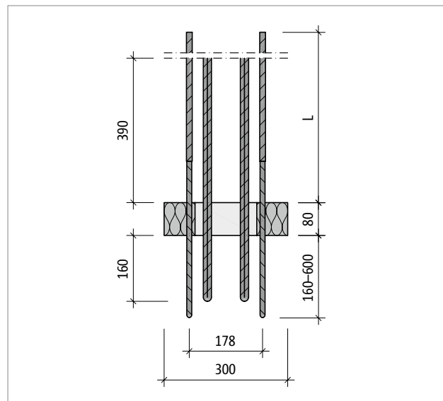
Abb. 188: Schöck Sconnex® Typ W-N1T1-V1H1-BW: Produktschnitt B-B
