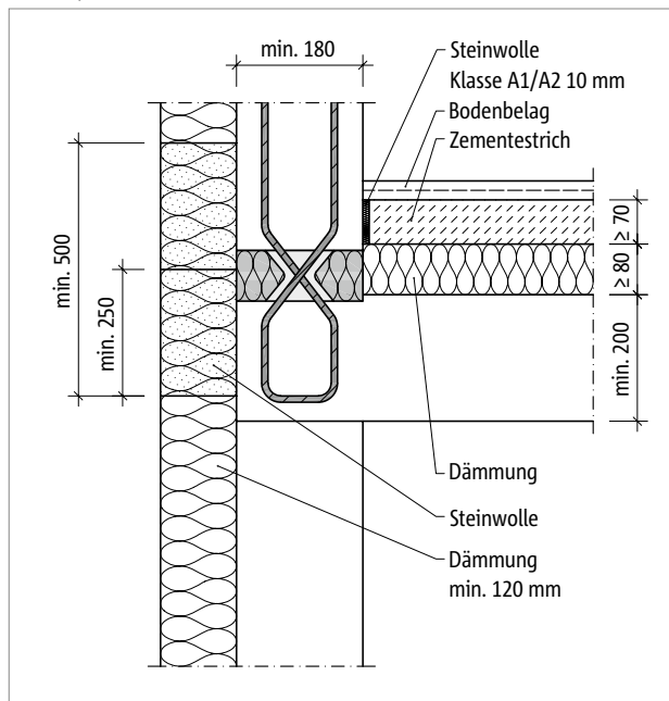
Abb. 206: Schöck Sconnex® Typ W-N-VH: Bei brennbarem WDVS mit Brandriegel aus Steinwolle
