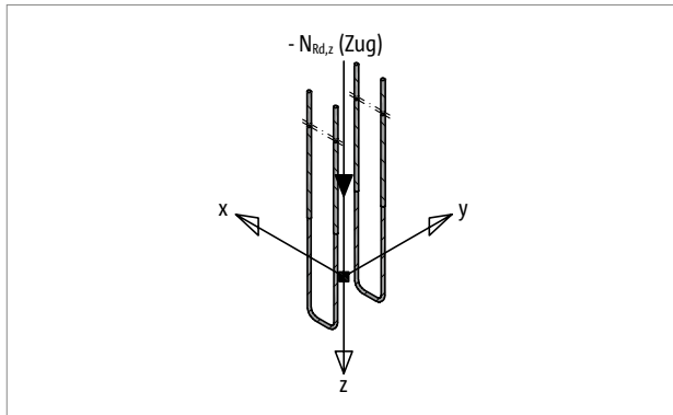
Abb. 161: Schöck Sconnex® Typ W-T: Die Bemessungskraft -N_{Rd,z} (Zug) im Koordinatensystem
