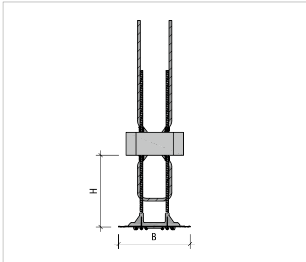
Abb. 198: Schöck Sconnex® Typ W: Produktschnitt mit Montagehilfe
