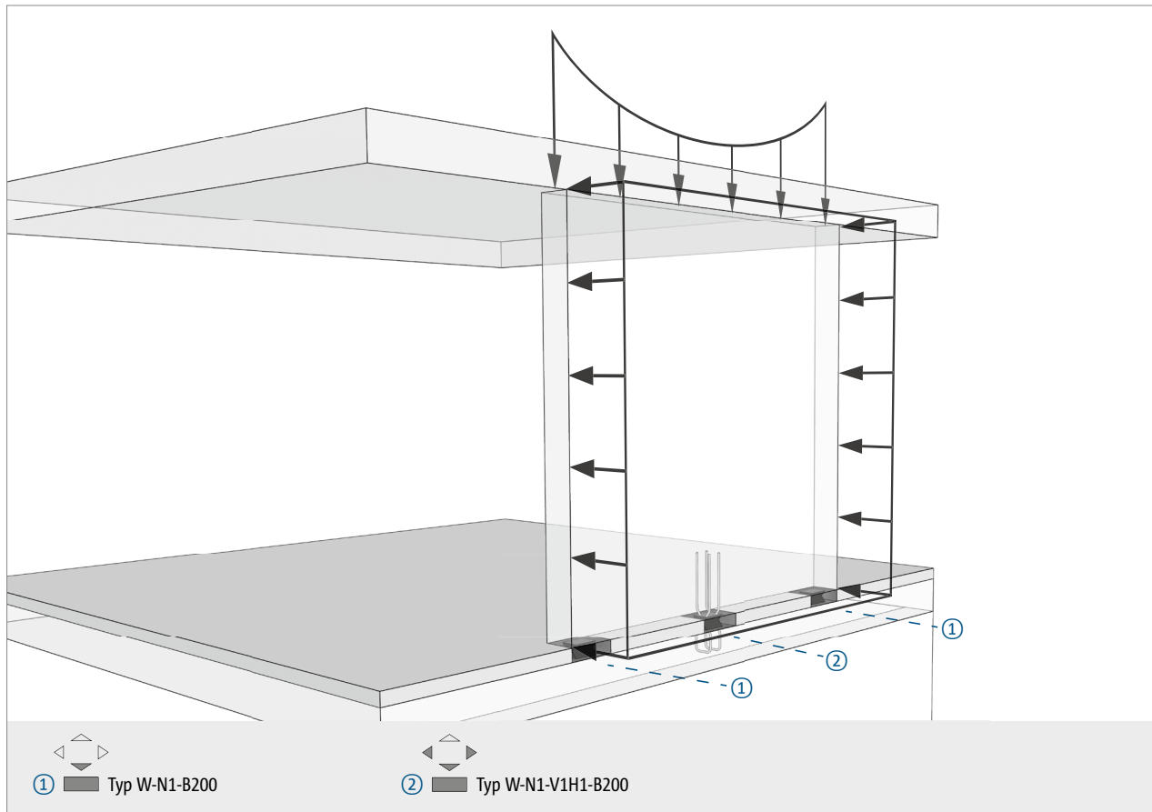
Abb. 153: Windbelastete Fassade wand auf der Decke getrennt
