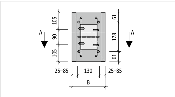
Abb. 185: Schöck Sconnex® Typ W-N1T1-V1H1: Produktgrundriss
