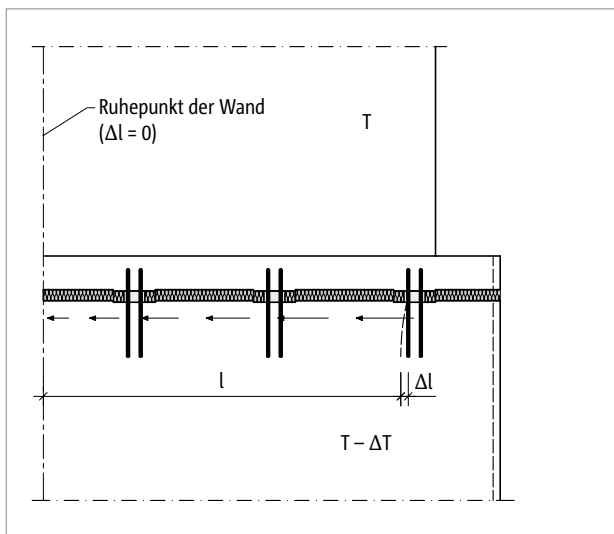
Abb. 170: Schöck Sconnex® Typ W: Verschiebung der äußeren Stäbe um \Delta l , bei Unterdeckendämmung infolge einer Abkühlung der Wand
