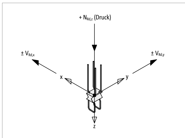
Abb. 164: Schöck Sconnex® Typ W-N-VH: Die Bemessungskräfte +N_{Rd,z} (Druck), +V_{Rd,x} und -V_{Rd,y} im Koordinatensystem
