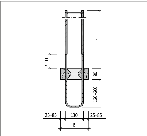
Abb. 181: Schöck Sconnex® Typ W-NT1T1-BW: Produktschnitt A-A
