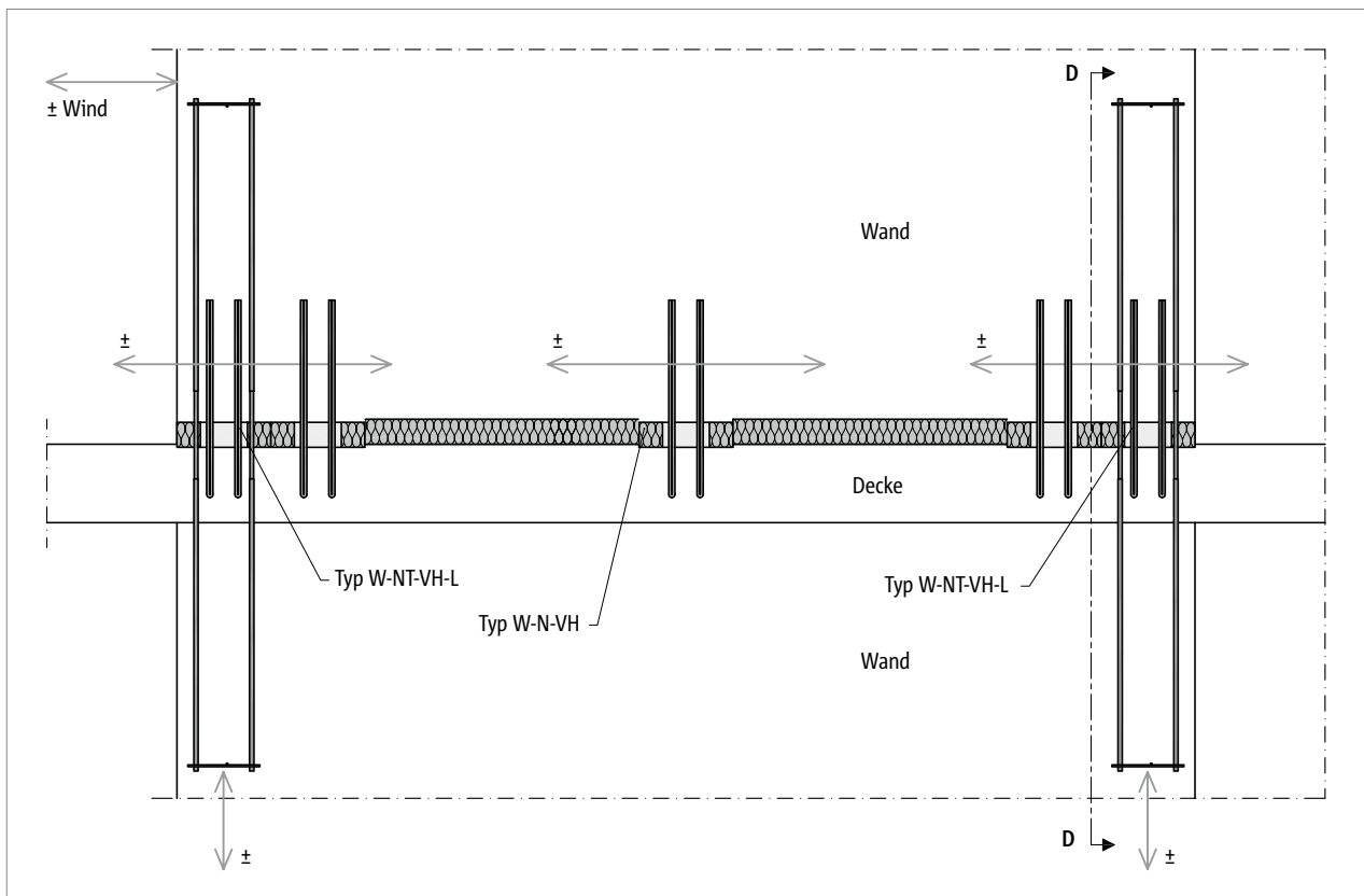
Abb. 143: Schöck Sconnex® Typ W: Kombinierte Produktvarianten für den Anschluss einer horizontal belasteten, stabilisierenden Wand
