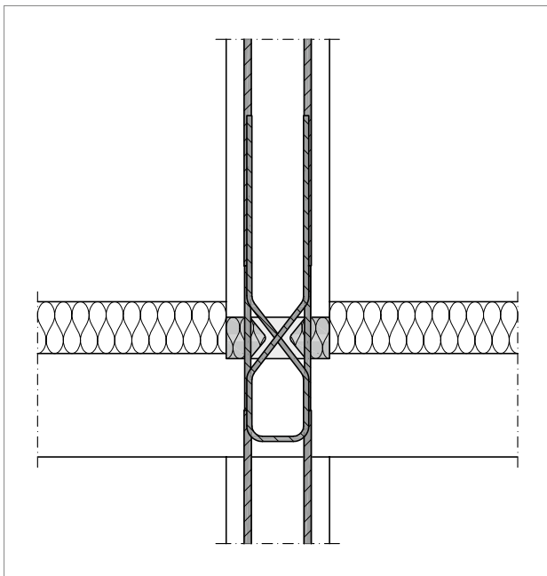
Abb. 145: Schöck Sconnex® Typ W-NT-VH-L: Schnitt D-D; Zugkraftverbindung der Wände durch die Decke hindurch
