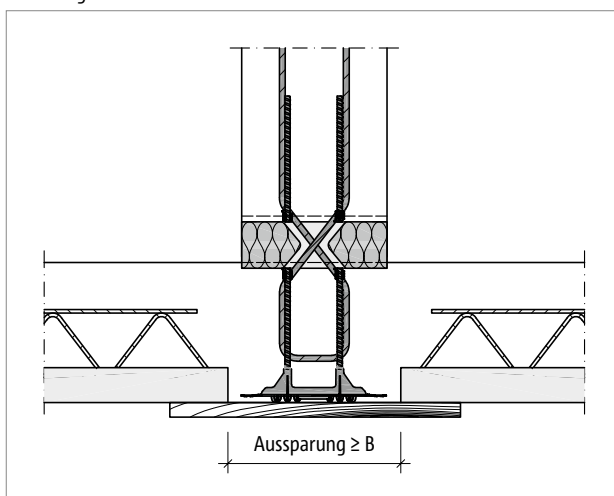
Abb. 244: Schöck Sconnex® Typ W: Schematische Darstellung (Einbaustand) Schöck Sconnex® Typ W bei Halbfertigteildecken und Aufdeckendämmung
