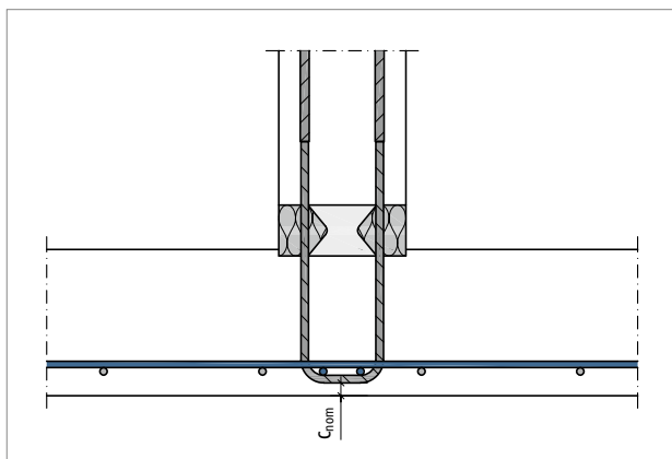
Abb. 162: Schöck Sconnex® Typ W-N1T1-BW: Die erste Deckenlage ist in den Schöck Sconnex® Bügel eingefädelt
