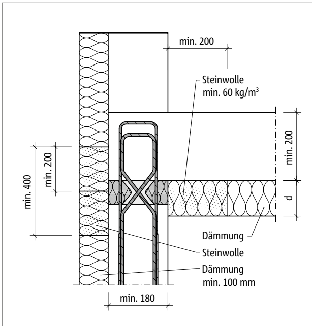
Abb. 220: Schöck Sconnex® Typ W-NT-VH: Bei brennbarem WDVS mit Brandriegel (außen) und Randstreifen aus Steinwolle (innen); Feuerwiderstandsklasse abhängig von der Dicke des Randstreifens
