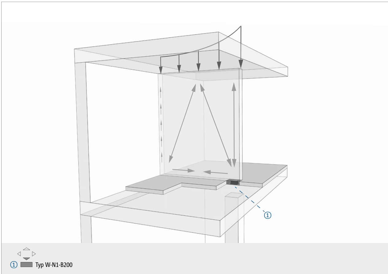
Abb. 155: Wand an Treppenhaus auf der Decke getrennt, punktuell gestützt
