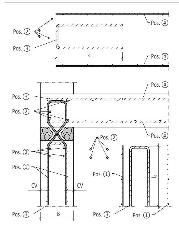
Abb. 231: Schöck Sconnex® Typ W-N-VH: Variante B – bauseitige Bewehrung für Anschluss am Wandkopf
