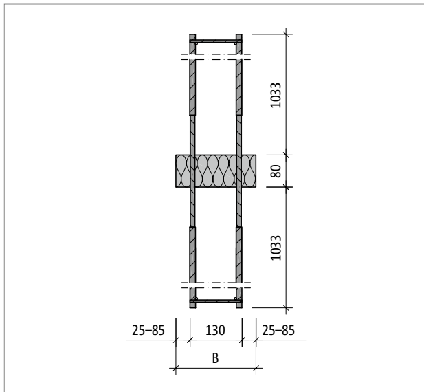
Abb. 195: Schöck Sconnex® Typ W-T1-LW: Produktschnitt A-A
