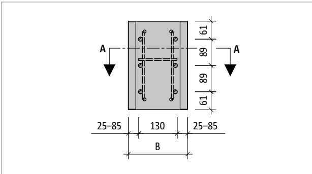
Abb. 191: Schöck Sconnex® Typ W-T2: Produktgrundriss
