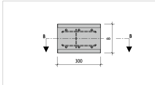
Abb. 192: Schöck Sconnex® Typ W-T2: Produktgrundriss
