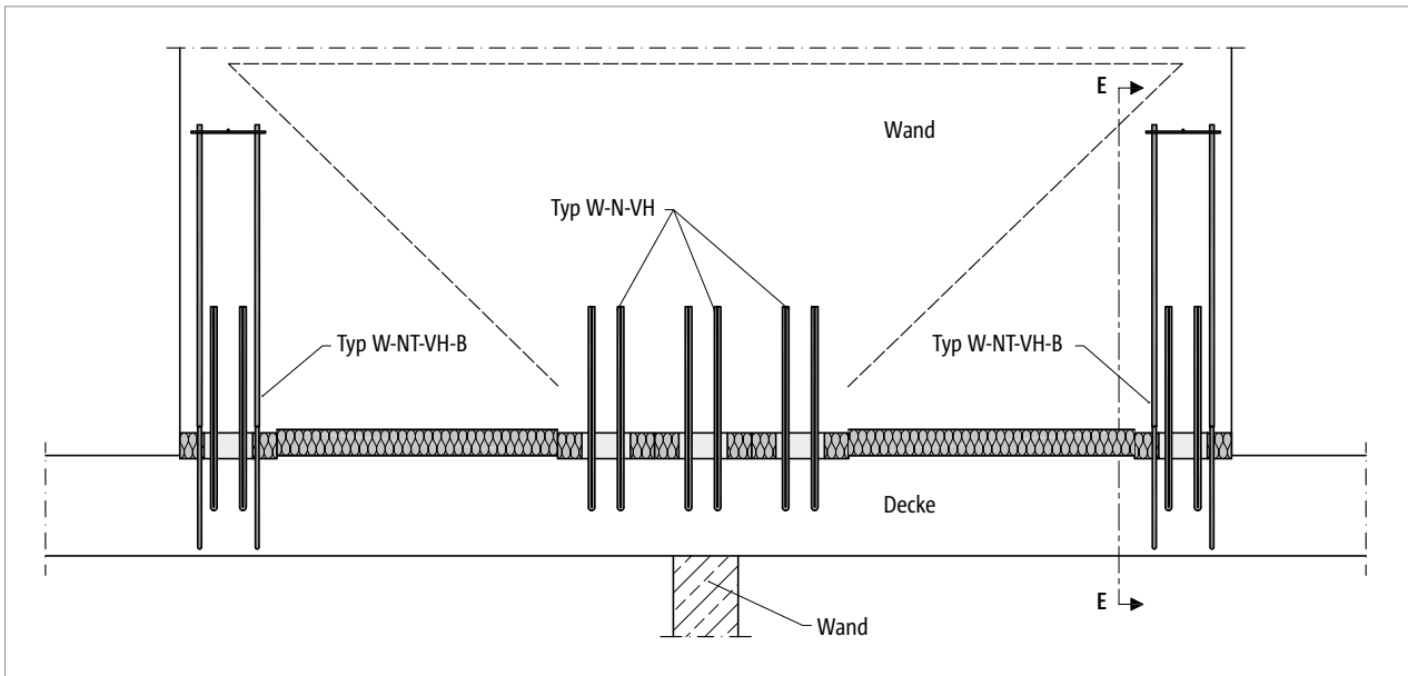
Abb. 144: Schöck Sconnex® Typ W: Kombinierte Produktvarianten im Anwendungsfall sich kreuzender Wände
