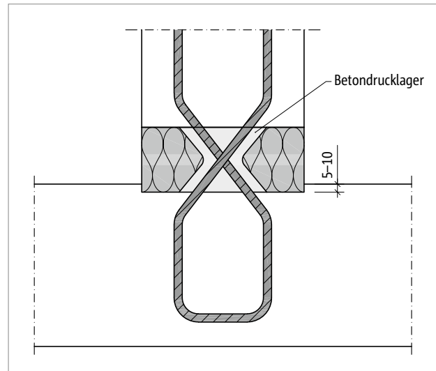
Abb. 238: Schöck Sconnex® Typ W: Detail 1; Formschluss durch 5–10 mm tiefe Einsenkung des Dämmkörpers in die Decke
