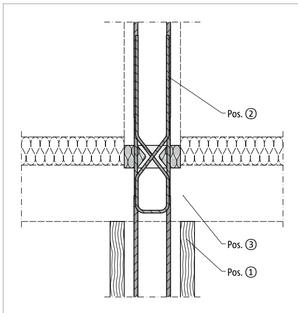
Abb. 241: Schöck Sconnex® Typ W-NT-VH-L: Einbau des Typ W mit Leistungsmerkmal T und Formvariante L für die Aufdeckendämmung in die Wand unter der Decke
