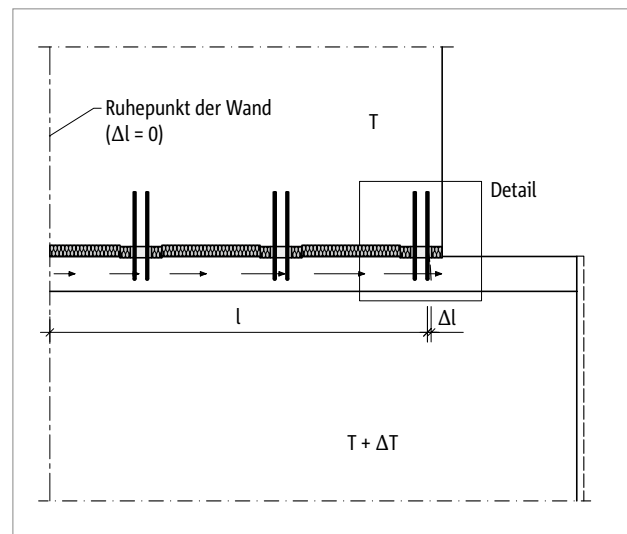
Abb. 171: Schöck Sconnex® Typ W: Verschiebung der äußeren Stäbe um \Delta l , bei Aufdeckendämmung infolge einer Erwärmung der Decke
