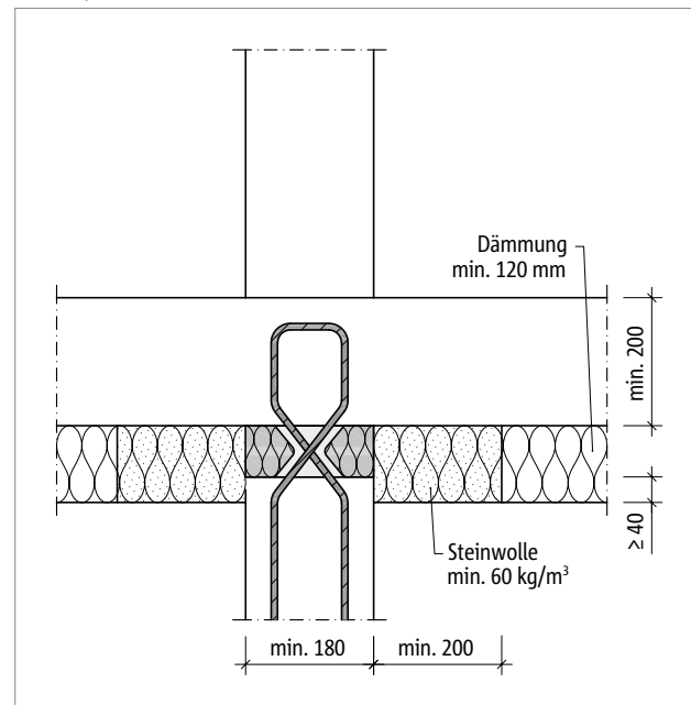
Abb. 208: Schöck Sconnex® Typ W-N-VH: Mit Randstreifen aus Steinwolle im Bereich der Unterdeckendämmung
