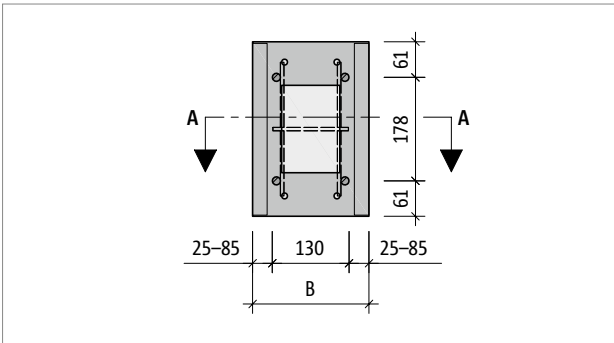
Abb. 179: Schöck Sconnex® Typ W-NT1T1: Produktgrundriss
