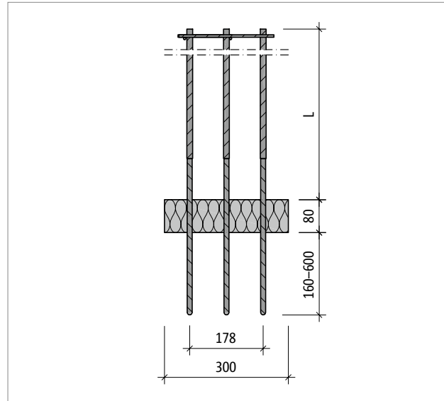
Abb. 194: Schöck Sconnex® Typ W-T2-BW: Produktschnitt B-B
