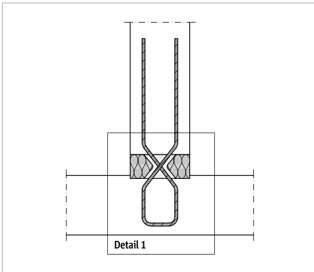
Abb. 237: Schöck Sconnex® Typ W: Formschluss zwischen der Oberkante der Decke und der Unterkante des Drucklagers ist sicherzustellen
