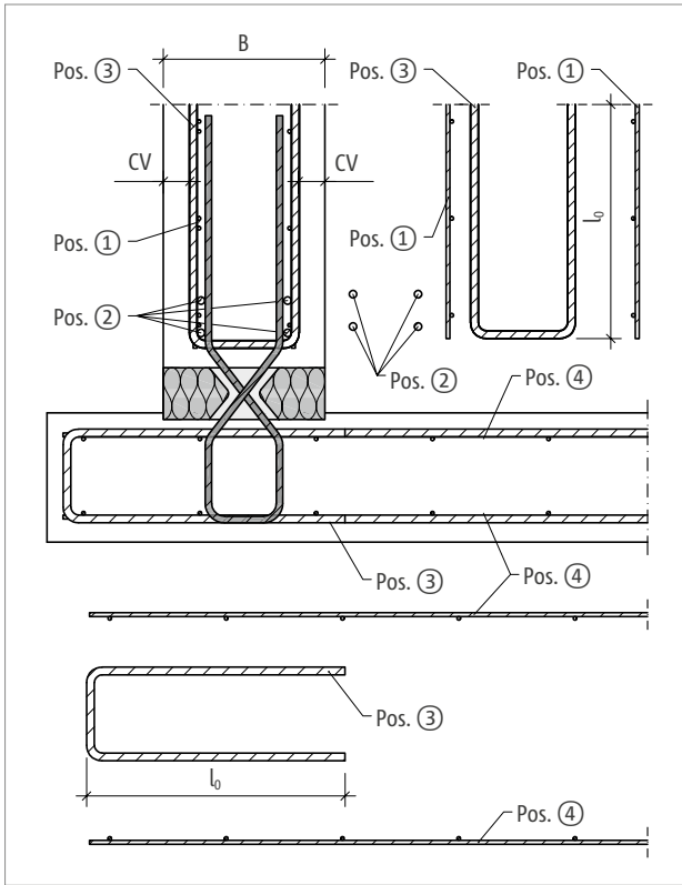
Abb. 228: Schöck Sconnex® Typ W-N-VH: Variante A – bauseitige Bewehrung für Anschluss am Wandfuß
