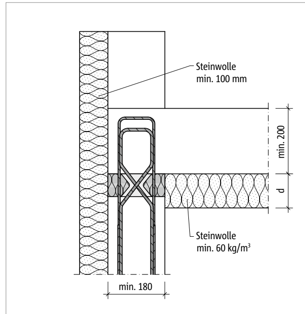
Abb. 221: Schöck Sconnex® Typ W-NT-VH: Bei nicht brennbarem WDVS (außen) und nichtbrennbarer Unterdeckendämmung aus Steinwolle (innen); Feuerwiderstandsklasse abhängig von der Unterdeckendämmung
