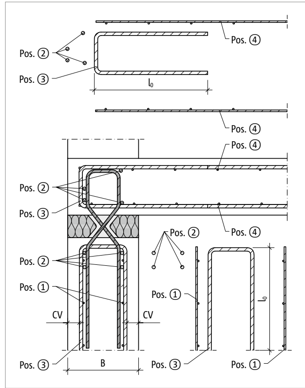
Abb. 229: Schöck Sconnex® Typ W-N-VH: Variante A – bauseitige Bewehrung für Anschluss am Wandkopf
