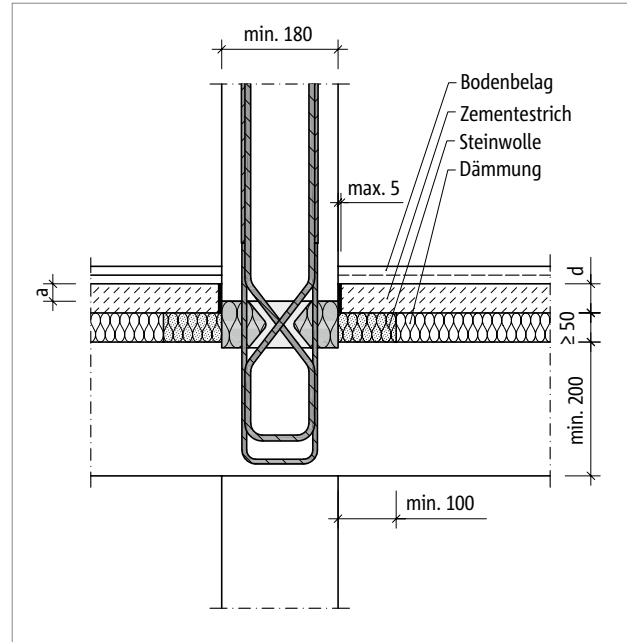
Abb. 214: Schöck Sconnex® Typ W-NT-VH: Mit Randstreifen aus Steinwolle im Bereich der Trittschalldämmung; Feuerwiderstandsklasse abhängig von der Estrichdicke
