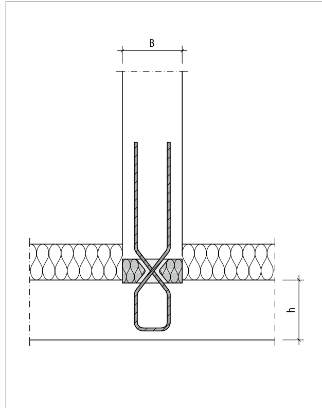
Abb. 246: Schöck Sconnex® Typ W-N-VH: Geometrie
