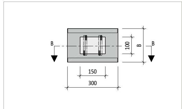
Abb. 176: Schöck Sconnex® Typ W-N-VH: Produktgrundriss; Drucklagerfläche 150 × 100 mm
