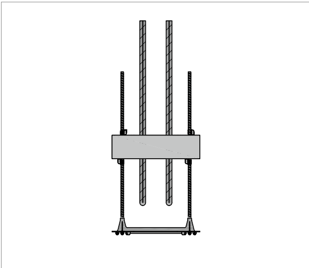
Abb. 197: Schöck Sconnex® Typ W: Produktansicht mit Montagehilfe
