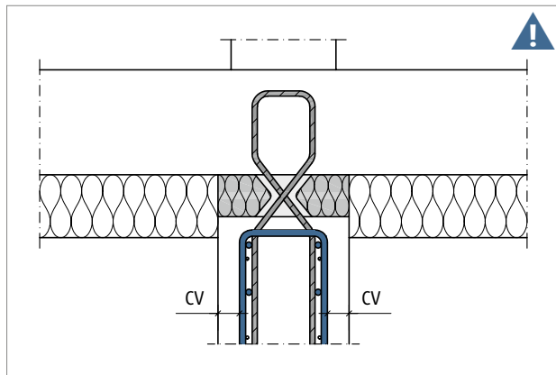
Abb. 165: Schöck Sconnex® Typ W-N-VH: Variante A – bauseitige Bewehrung; die außenliegende Längsbewehrung stützt die Querkraftstäbe des Schöck Sconnex® gegen die Bauteiloberfläche ab
