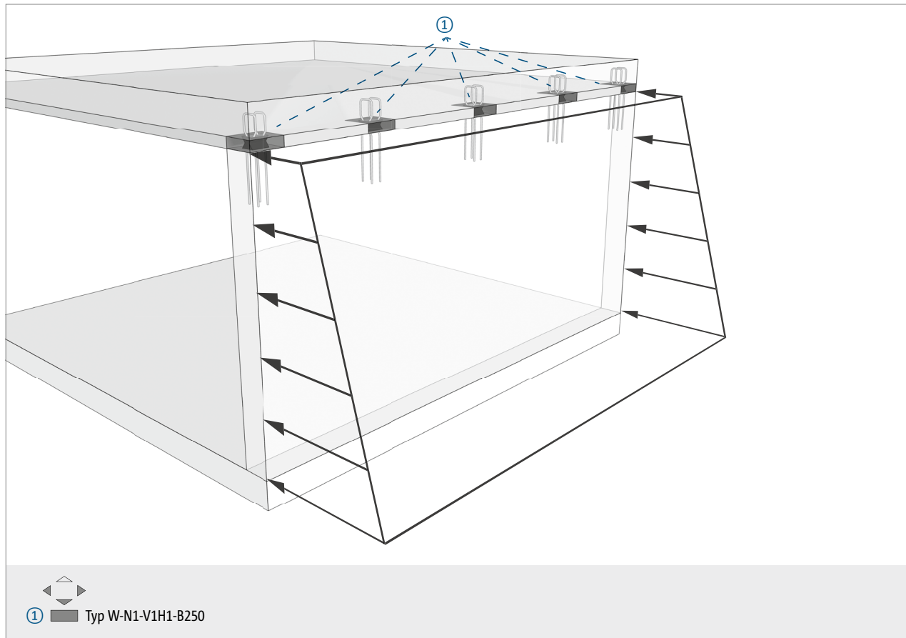
Abb. 152: Erddruckbelastete Wand unter Decke getrennt
