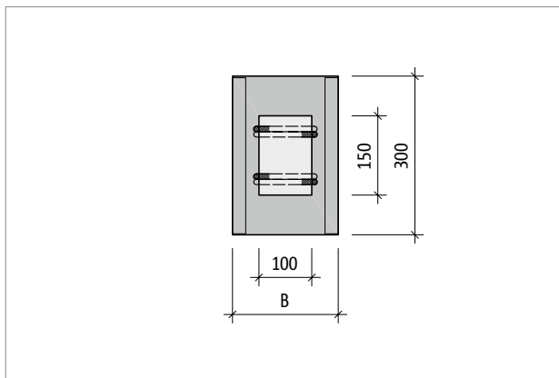
Abb. 167: Schöck Sconnex® Typ W-N-VH: Produktgrundriss; Drucklagerfläche 150 mm × 100 mm
